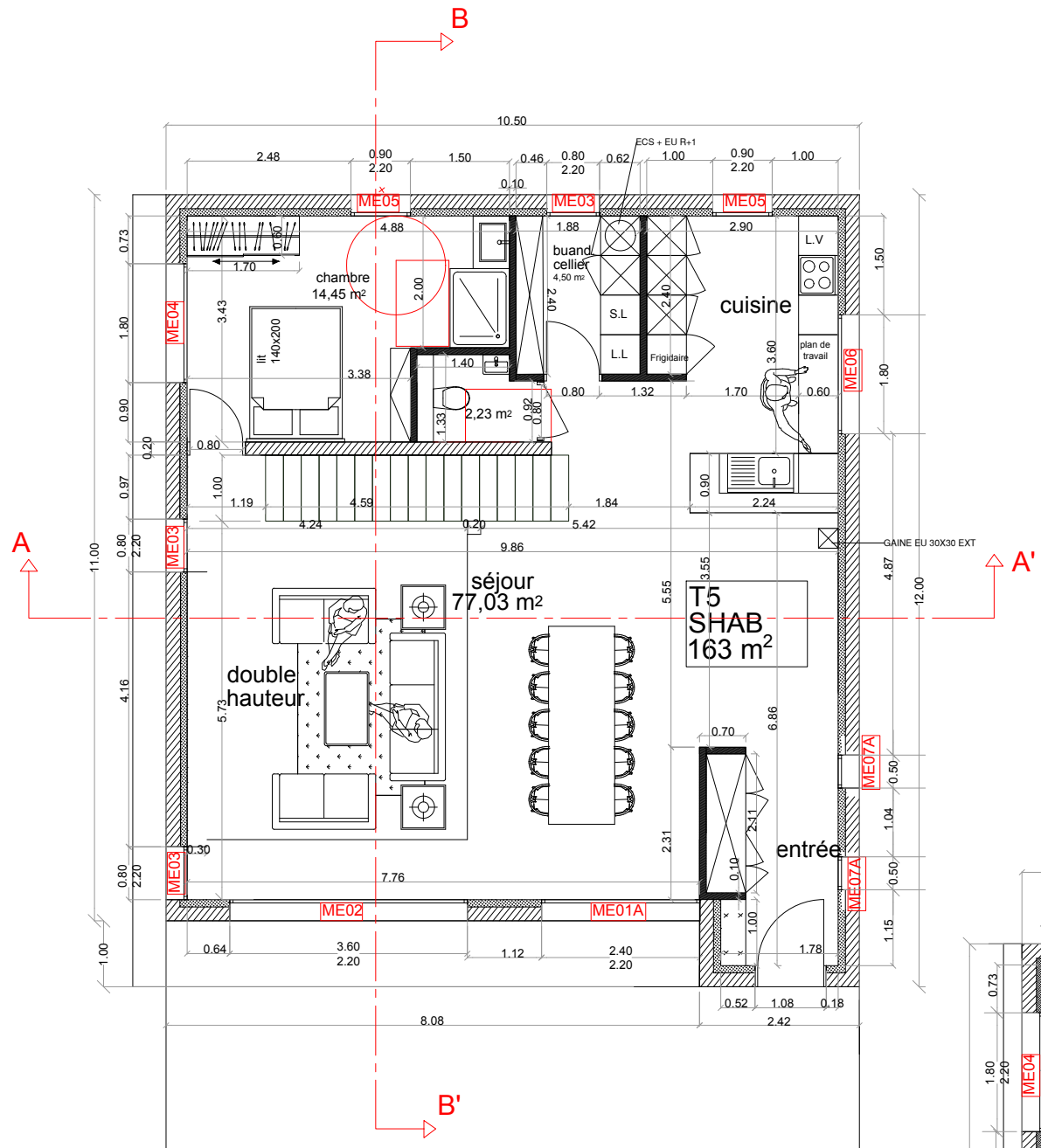
villa Type 1a RDC
